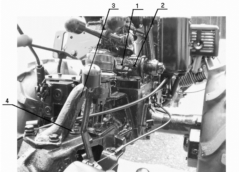
Рисунок 10 – Тяга рулевого управления
