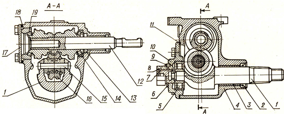
Рисунок 11 Рулевой механизм
